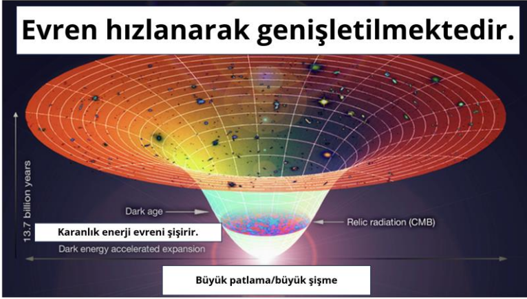
Resim 2: Evren karanlık enerji tarafından hızlanarak genişletilmektedir.
