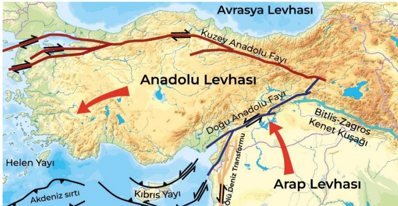
Resim 58: Arap levhası Anadolu levhasını batıya doğru itmektedir
